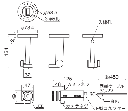
外形寸法図 (単位: mm)
